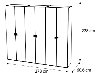
6 door wardrobe
